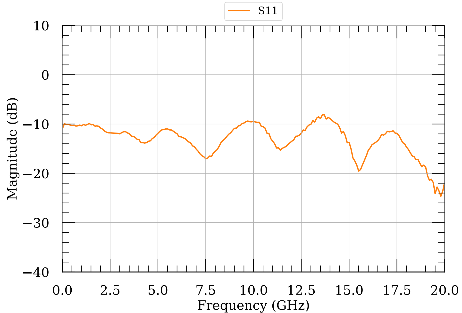
LNA S-params module028v2
